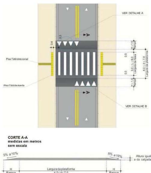
Figura 29. Especificações para as travessias elevada
