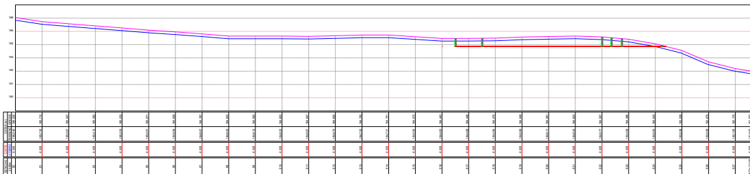
Perfil Longitudinal 01
