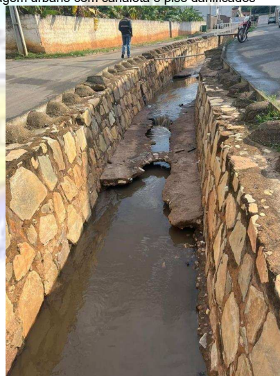
Imagem 09 – Trecho de canal de Drenagem urbano com parede, canaleta e piso danificados
