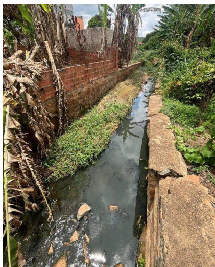
Imagem 8 – Trechos de canal de Drenagem urbano com canaleta e piso danificados
