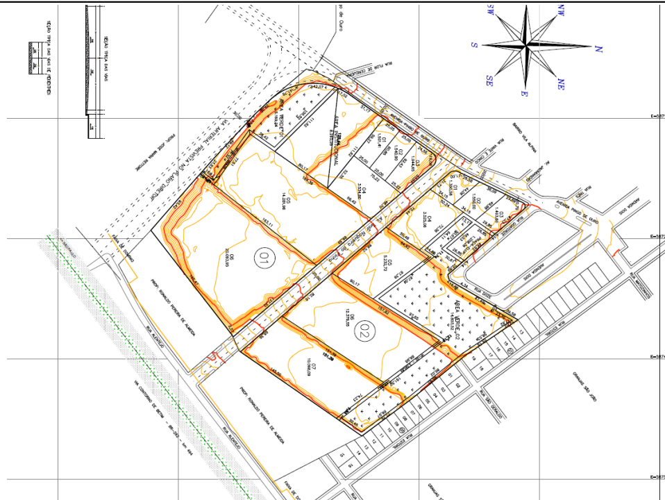
Figura 11 - Recorte da Planta com Taludes, apresentado pelo RT.
