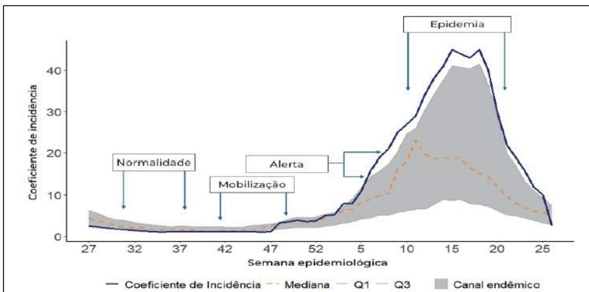
Figura 1 – Exemplo de estruturação de diagrama de controle e seus componentes (canal endêmico, mediana, taxa de incidência)
