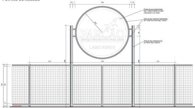
ANEXO IV PORTÃO DE ACESSO
