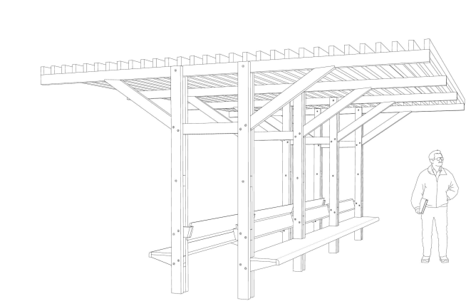
ANEXO V MODELO DE PERGOLADO - Legendas e Notas
