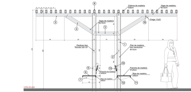
ANEXO V MODELO DE PERGOLADO - Corte longitudinal
