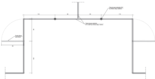
ANEXO IV PORTÃO DE ACESSO - Planta baixa
