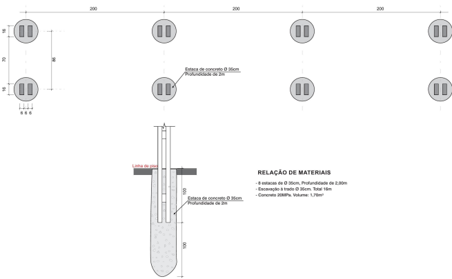
ANEXO V MODELO DE PERGOLADO - Pilares e estacas
