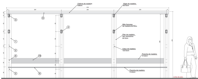
ANEXO V MODELO DE PERGOLADO - Pilares e estacas
